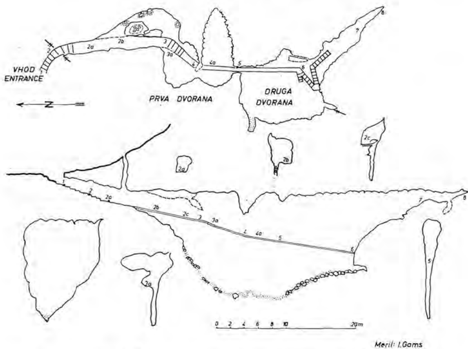
Sl. 1. Železna jama, tloris, naris in prečni profili
